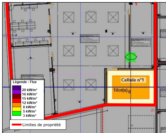
Figure 5. Représentation graphique effets thermiques générés par un incendie sur le stockage des caisses vides
