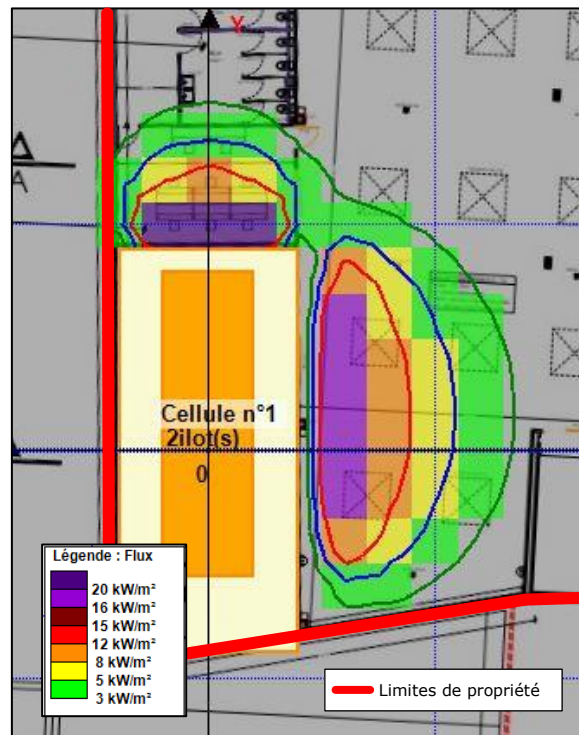
Figure 2. Représentation graphique effets thermiques générés par un incendie sur le stockage frigorifique de matières premières
