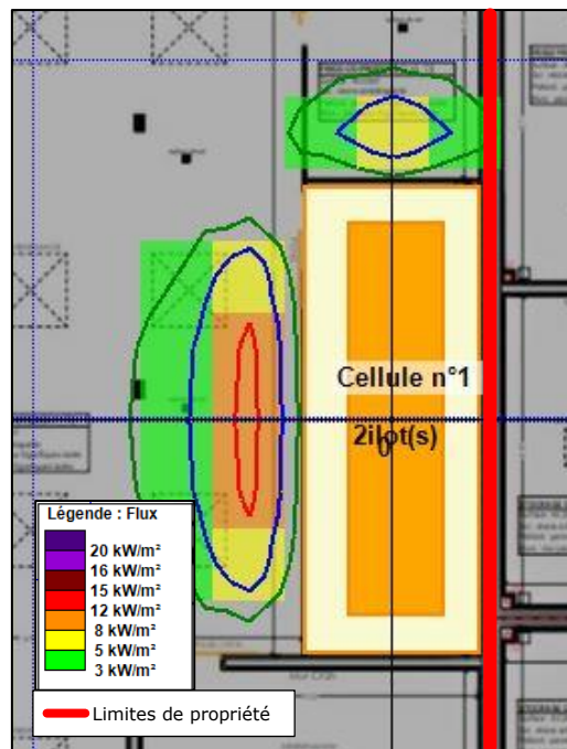
Figure 4. Représentation graphique effets thermiques générés par un incendie sur le stockage des produits finis
